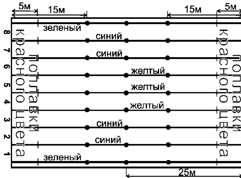
Рисунок 1. Схема расположения разделительных дорожек
